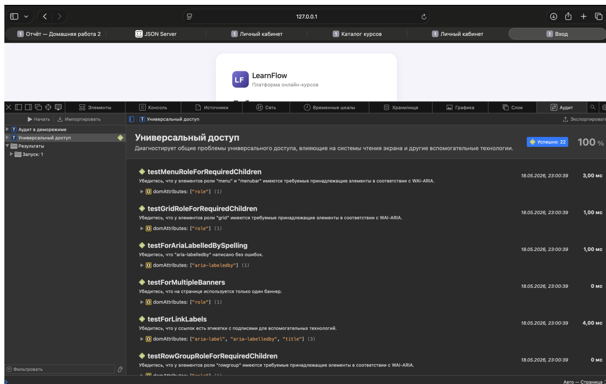
Рис. 1: Аудит универсального доступа — login.html
